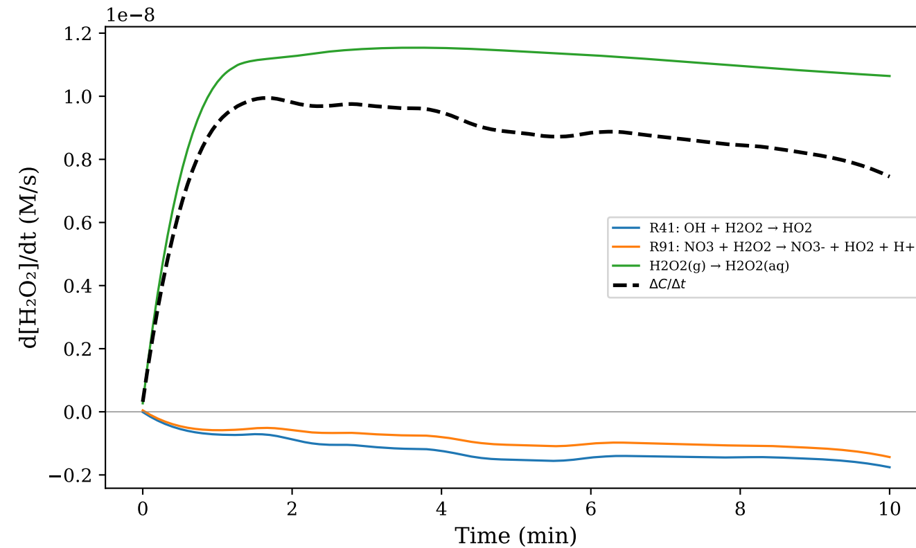
(d) \text{H}_2\text{O}_2
